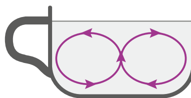
2. При размешивании воды в чашке ложечкой в жидкости образуются вертикальные вихри
