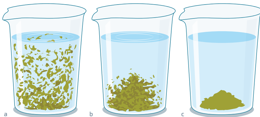
3. Опыт Эйнштейна. Воду с чайинками размешивают ложечкой (а). Вскоре чайинки собираются в центре стакана (б) и в конечном итоге опускаются на дно (с). Их движение доказывает наличие вертикальных вихрей, хотя их существование, кажется, противоречит интуиции
