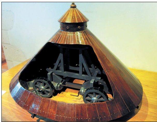
Танк Леонардо — современная реконструкция на основе дошедших до нас рисунков великого мастера
