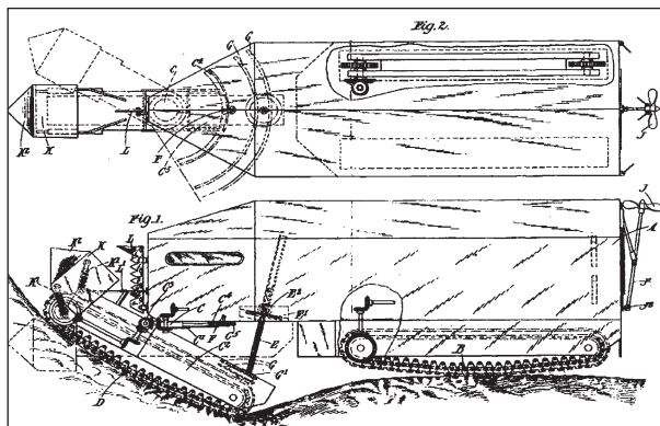
Схема амфибийного танка Макфая
